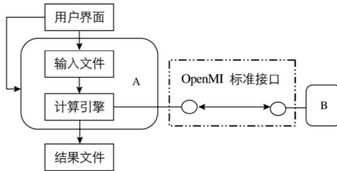
图3 OpenMI 标准接口原理
